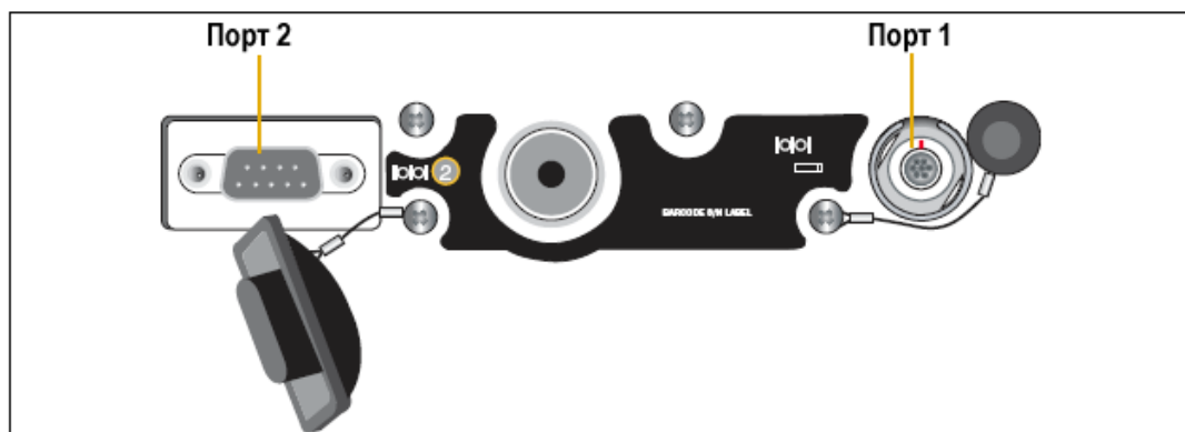
Рис. 8.1. Последовательные порты приемника
