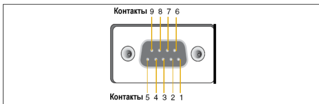
Рис. 8.3. Нумерация контактов разъема Порт 2.
