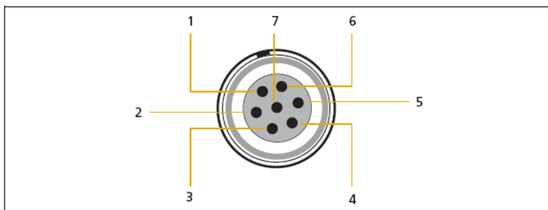
Рис. 8.2. Нумерация контактов разъема Порт 1.
