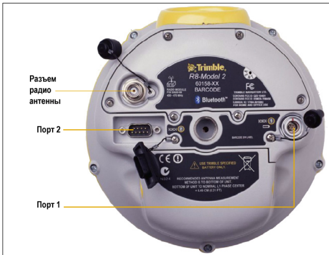
Рис. 2.2 Нижняя панель приемника Trimble R8 GNSS
