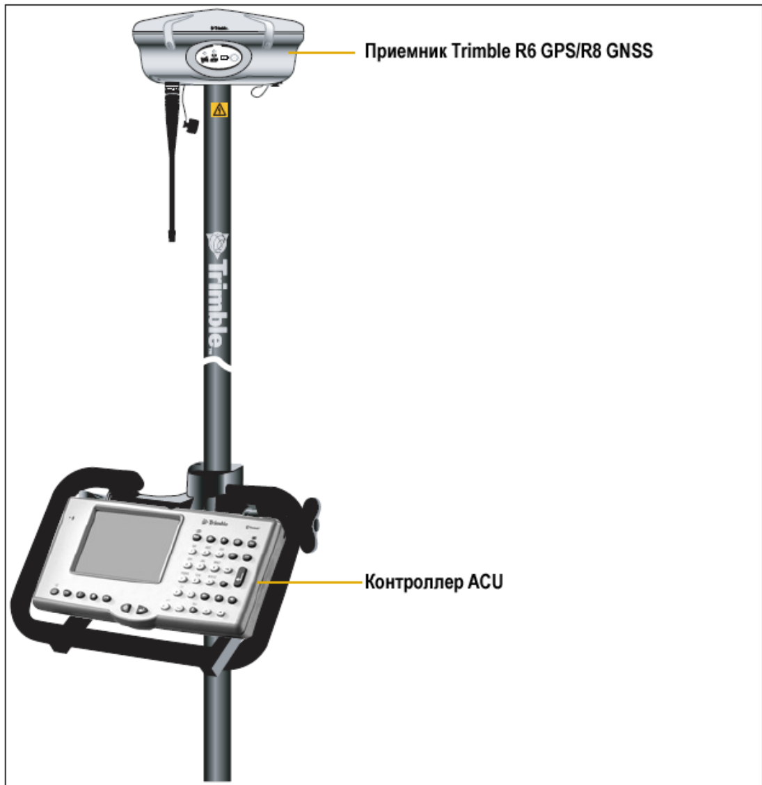
Рис. 2.3 Крепление приемника на вехе
